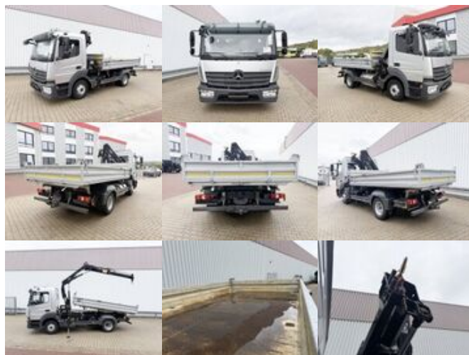
Mercedes-Benz Atego 1018 K 4x2 Atego 1018 K 4x2, 2x AHK, Kran Hiab 055 DS-1 Duo
