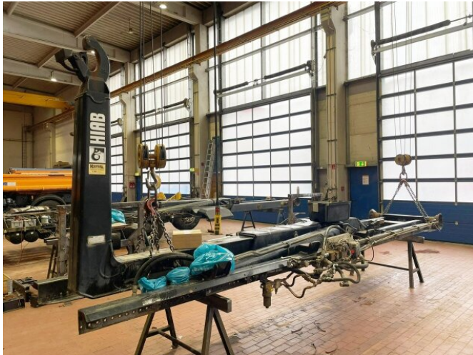
HIAB XR21S59 Abrollanlage XR21S59 Abrollanlage
