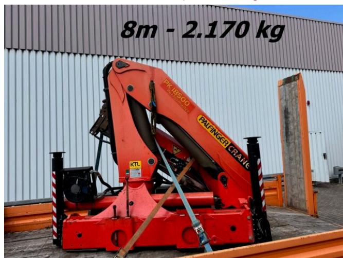
Palfinger PK 18500-A PK 18500-A
