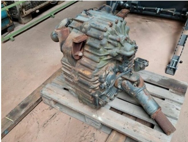
Mercedes-Benz MB Verteilergetriebe MB Verteilergetriebe
