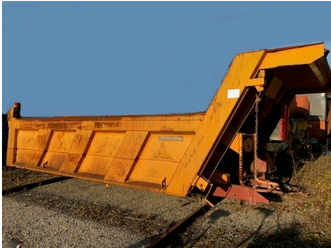
Meiller Mulde ca. 12,5m 3 Meiller Mulde, Jet Design ca. 12,5 cbm, Heckklappe, Dachschutz
